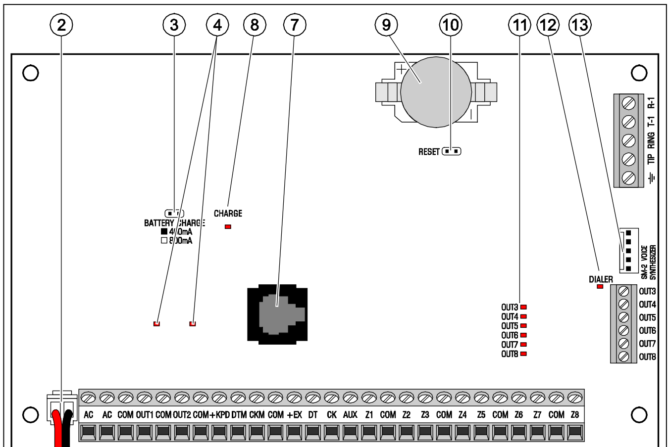
Rys. 3. Płyta główna centrali alarmowej INTEGRA 32 (wersja 1.4 F).
